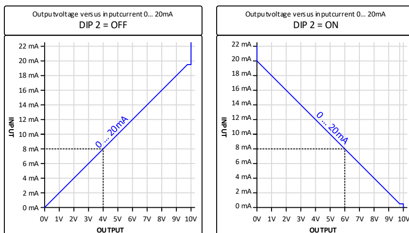
Figuur 6: Uitgang versus ingang
