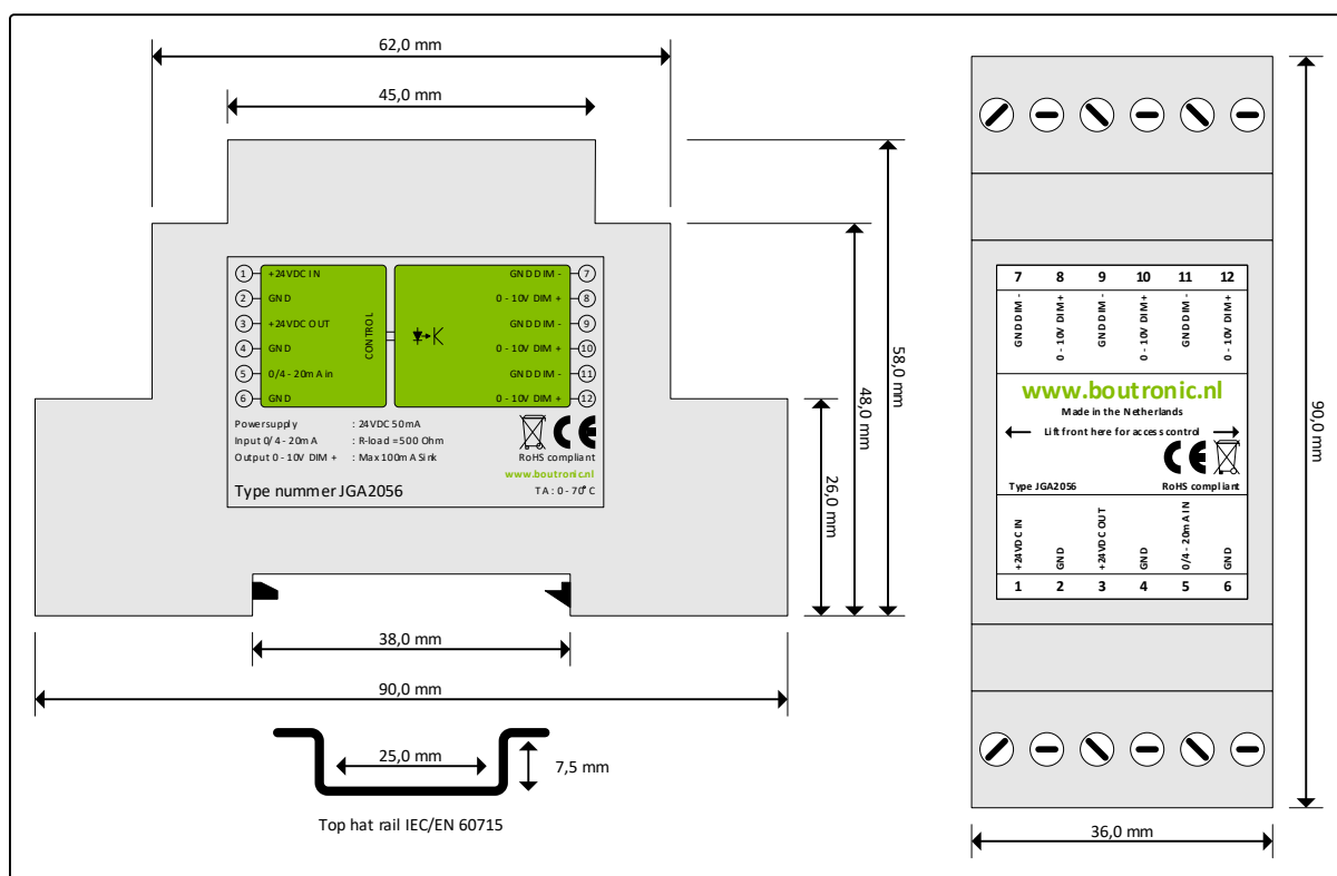
Figuur 8: Afmetingen
