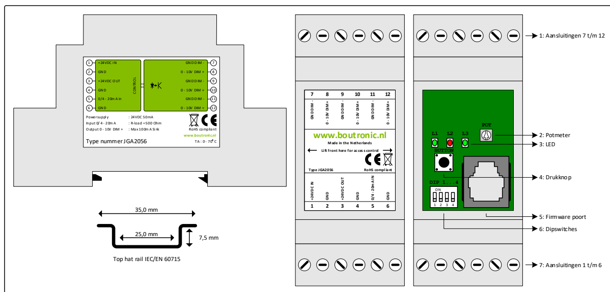
Figuur 1: Schematische weergave JGA2056
