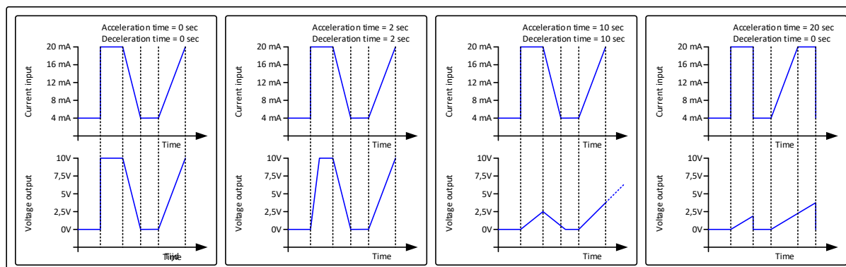
Figuur 7: voorbeeld stuurvertraging
